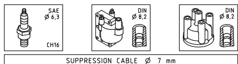
SUPPRESSION CABLE Ø 7 mm
