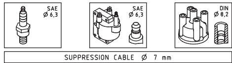
SUPPRESSION CABLE \varnothing 7 mm
