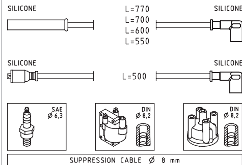
SUPPRESSION CABLE Ø 8 mm
